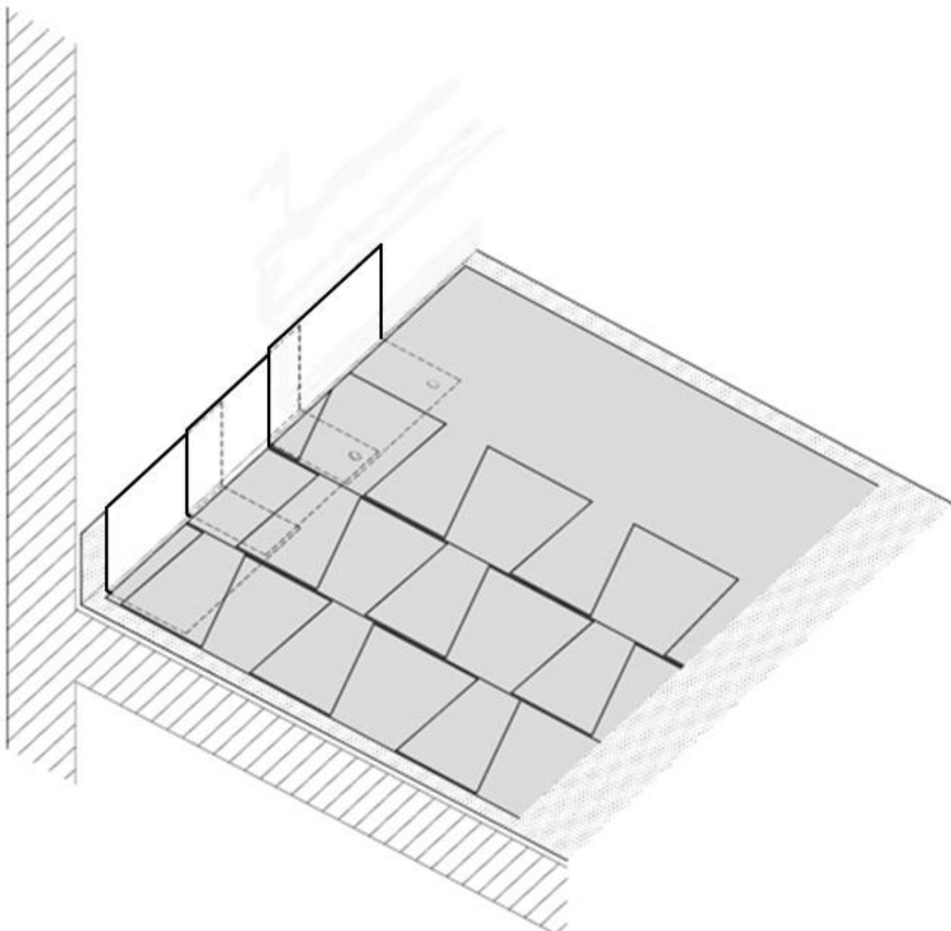
DIAGRAMA 5: DETALLE PARA INSTALAR VIERTEAGUAS ESCALONADOS CON VIERTEAGUAS DE REMATE
